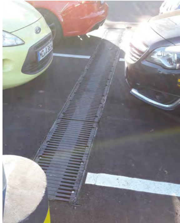
BIRCOpur® ist ständig einsehbar und leicht zu öffnen. Es können 20 m 2 vollversiegelte Fläche an einen Laufmeter Rinne angeschlossen werden. Foto: Müller + Huber
