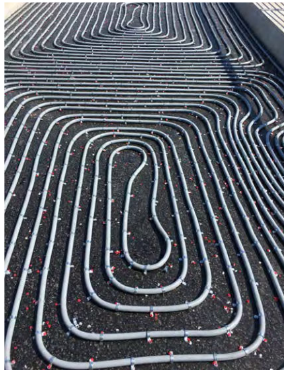
Bild 3: Installierte Heizschleifen auf der Tragschicht der Brücken in Ingolstadt.
