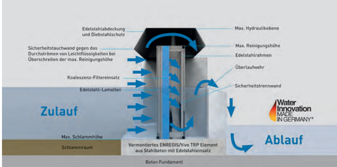
Funktionsbeschreibung ENREGIS/Vivo® TRP
