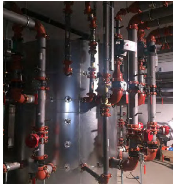
Das erste CO 2 -neutrale ICE-Instandhaltungswerk der Deutschen Bahn wird durch ein hochmodernes Kühlwasser-Heizsystem mittels Geothermie klimatisiert. Victaulic lieferte für die Bahn genutete Rohrkupplungen, Armaturen und Formteile. (Quelle: Victaulic)
