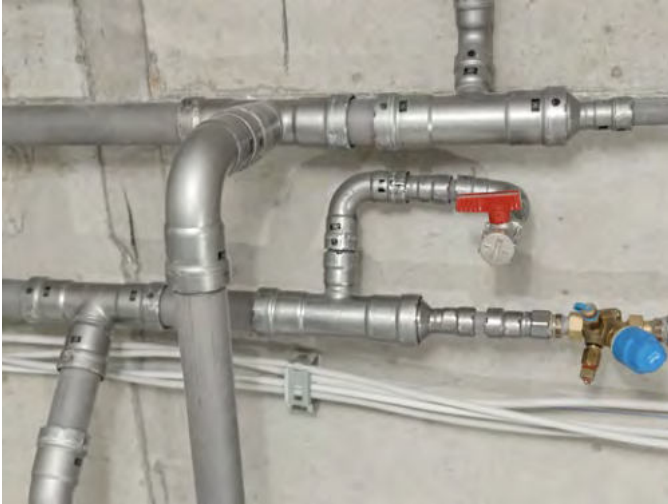
Durch die breite Palette an Formteilen erwies sich das „Megapress“-System als echter Problemlöser für die unterschiedlichsten Installationsaufgaben.
