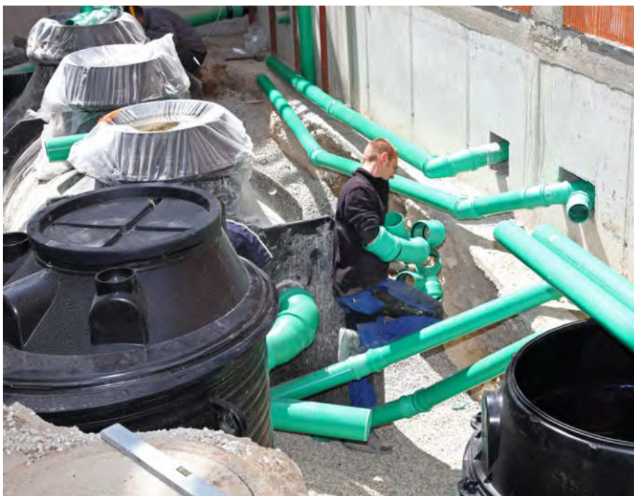
Bild 4: Die Hybrid-Hebeanlage ist dem eingebauten Wickelrohrabscheider nachgeschaltet. (Bild: KESSEL AG)
